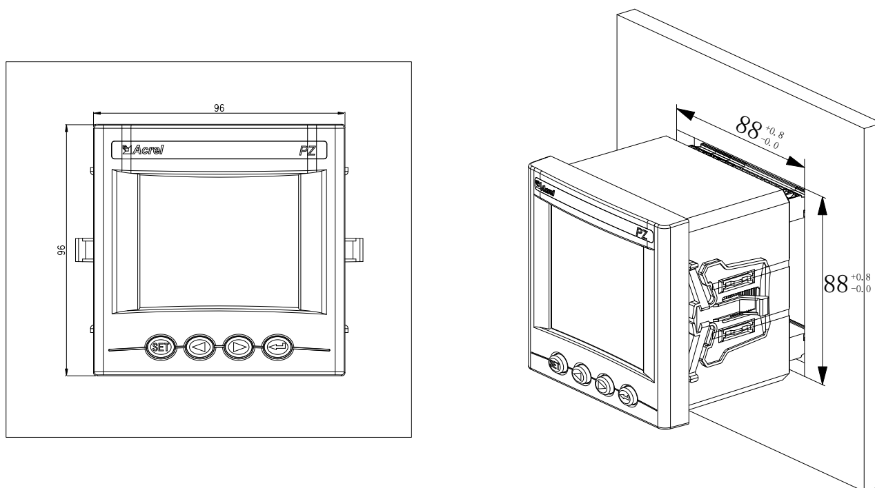
图 6 PZ96 安装尺寸
