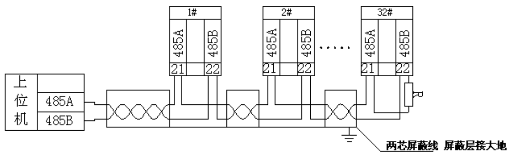
图 13 RS485 通讯接线示意图
