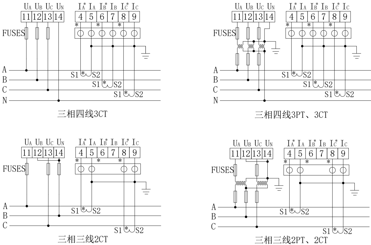
图 12 仪表信号接线示意图
