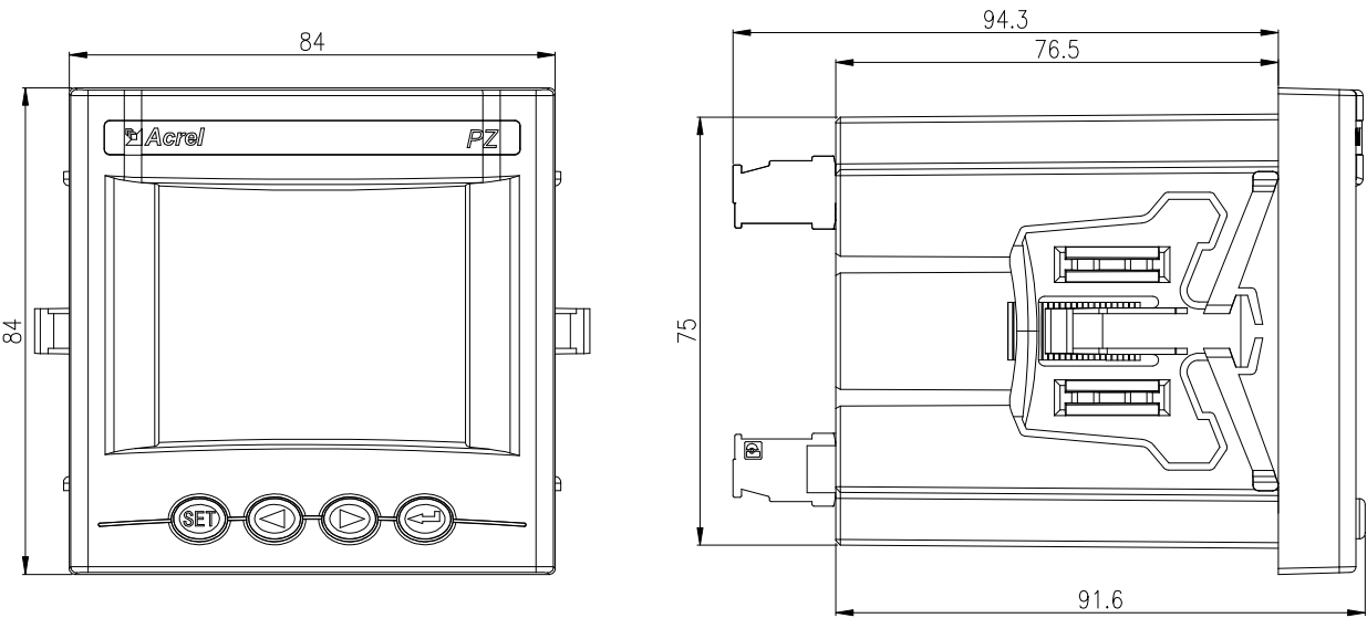
图 2 PZ80 外观尺寸
