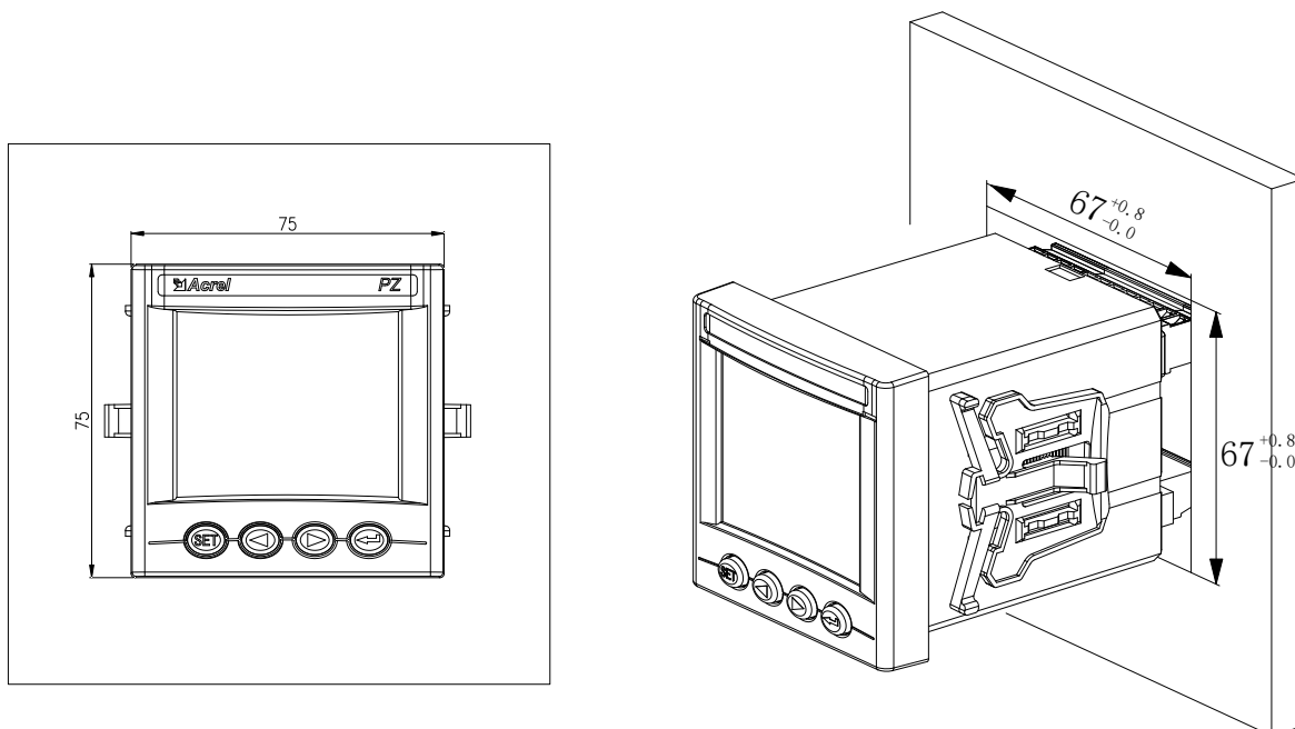
图 4 PZ72 安装尺寸
