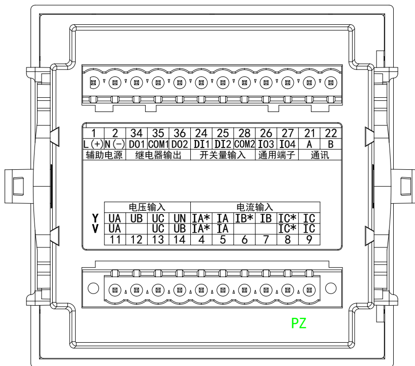
图 10 PZ80 系列接线端子图
