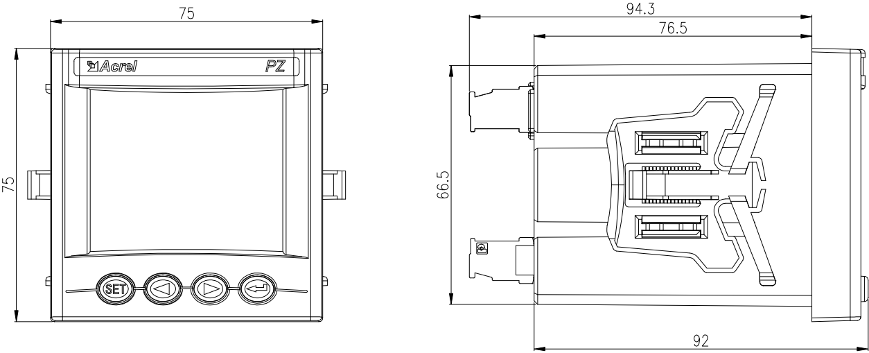
图 1 PZ72 外观尺寸
