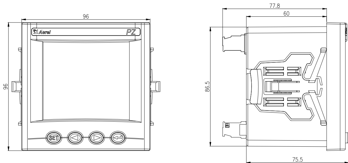
图 3 PZ96 外观尺寸
