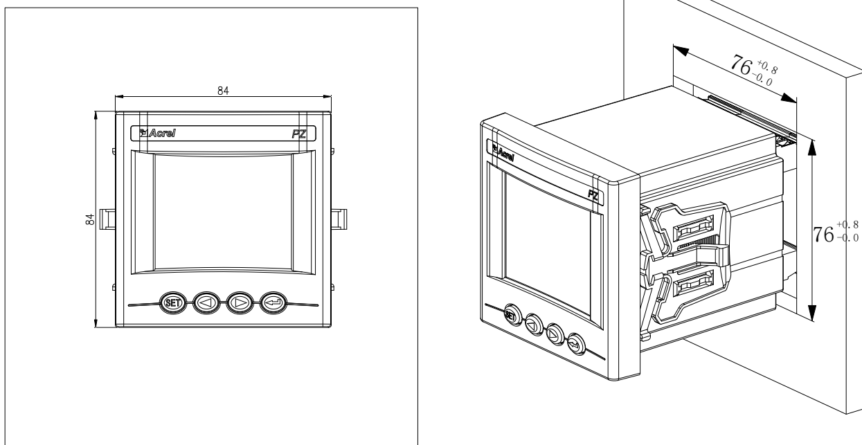
图 5 PZ80 安装尺寸
