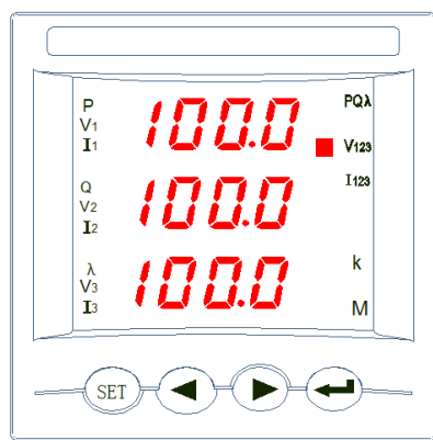
图 14 数码管显示前面板
