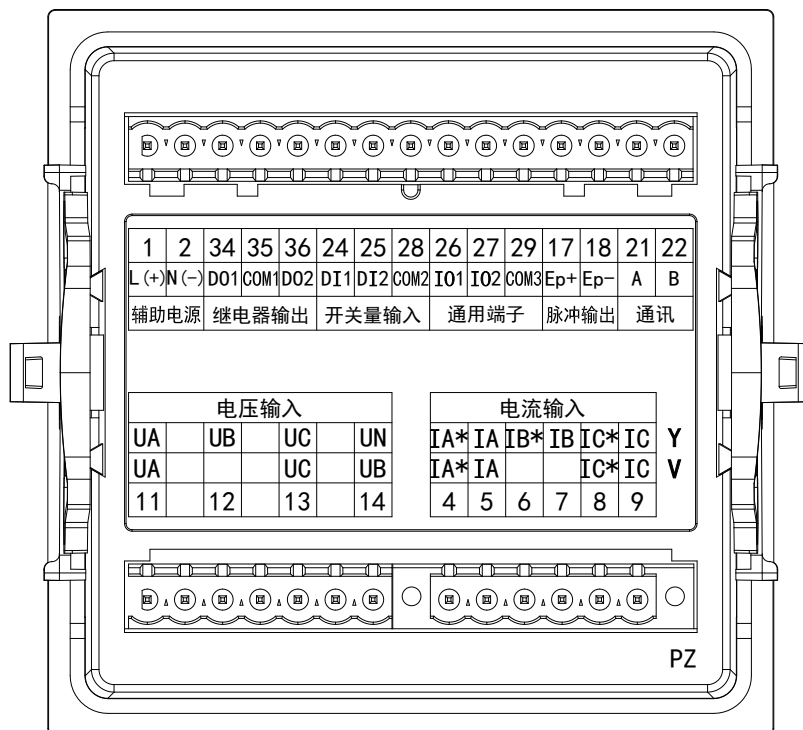
图 11 PZ96 系列接线端子图
