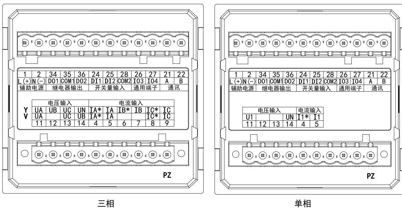
图 9 PZ72 系列接线端子图
